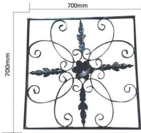
WPU0014 20mm x 5mm Flat Bar Dim - 700mm x 700mm
