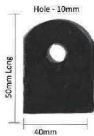
40x10 Flat Bar Lug 50mm Long x 40mm Wide
